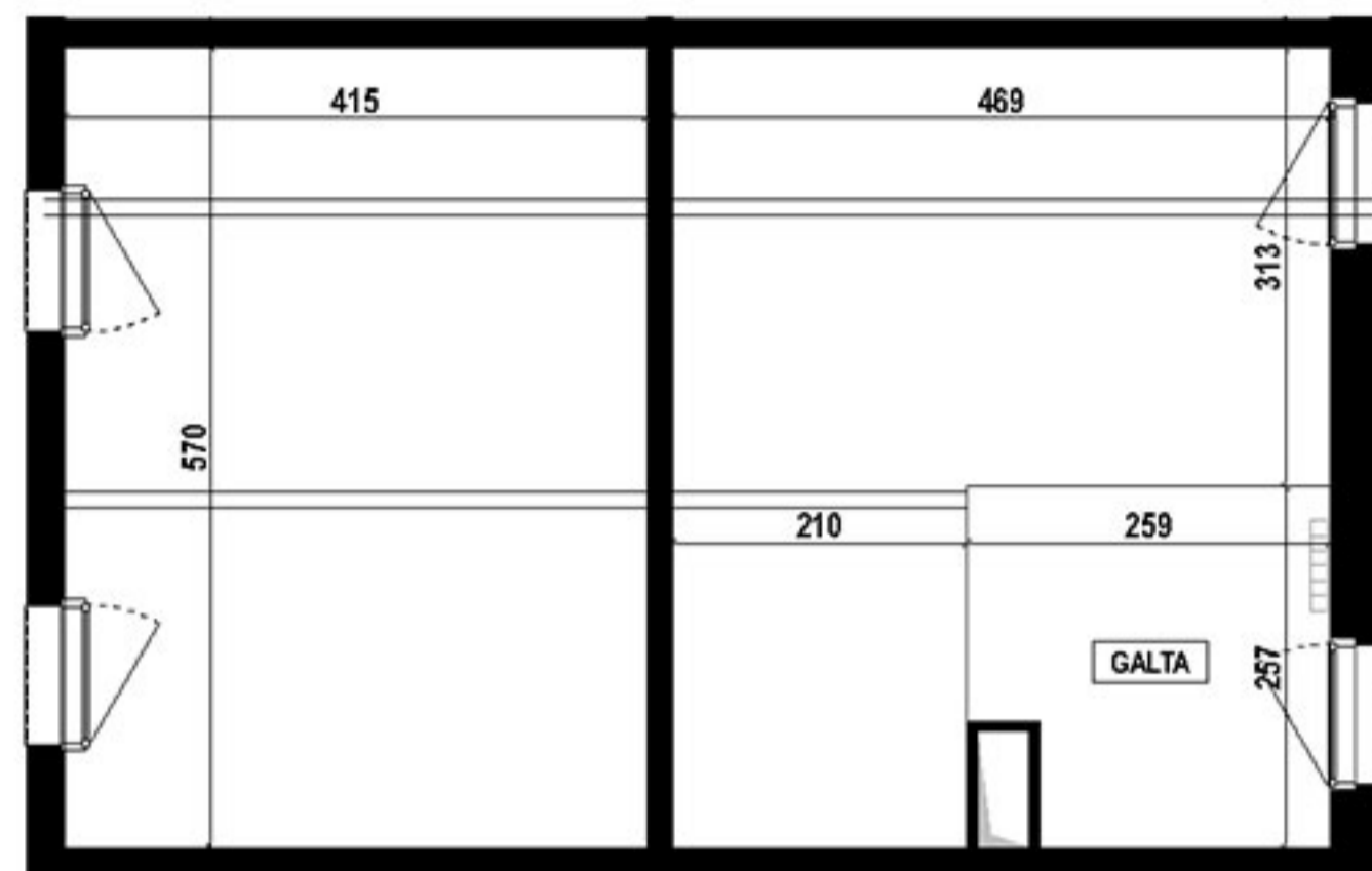
1 er ETAGE
