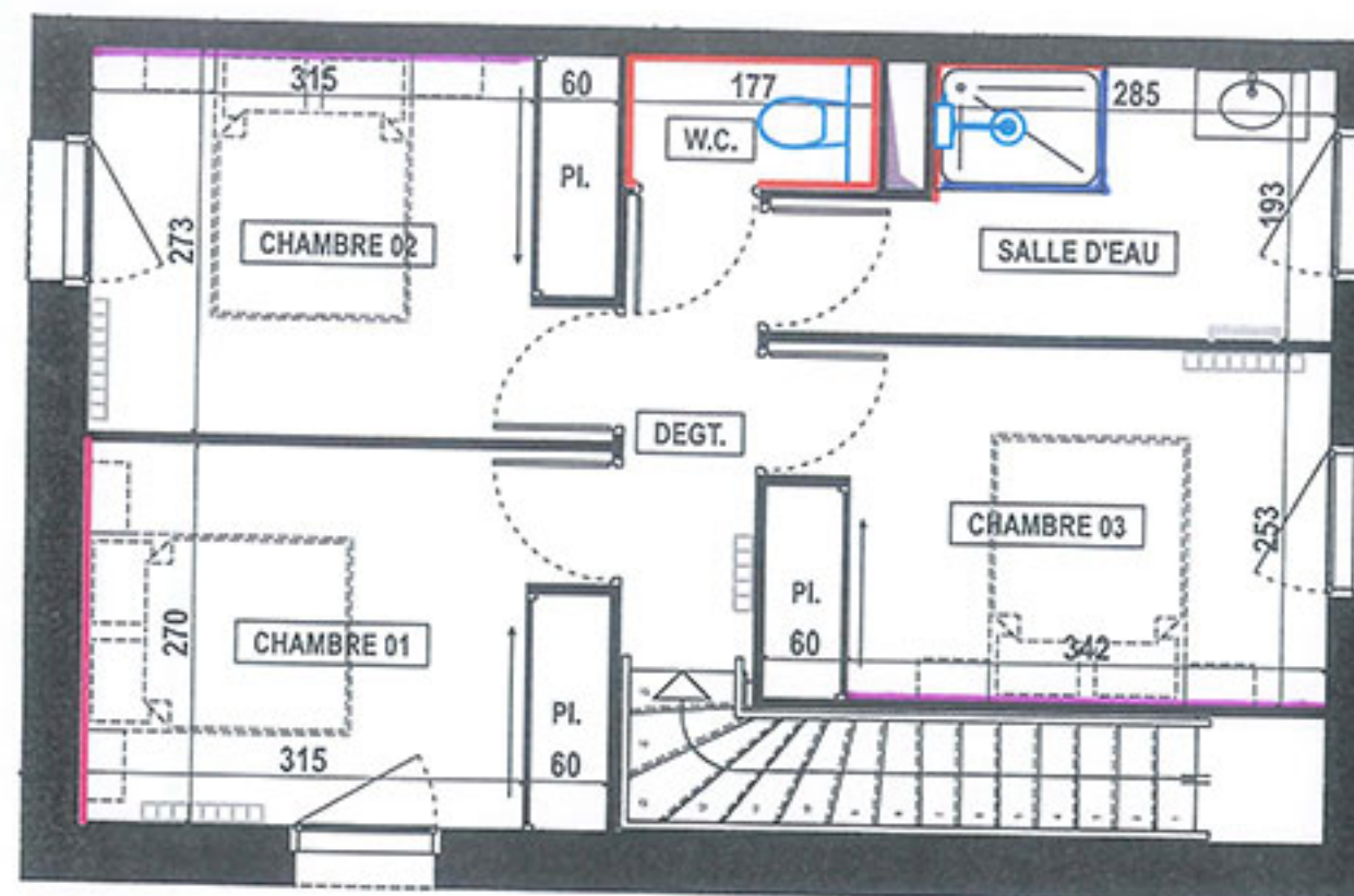
1 er ETAGE
