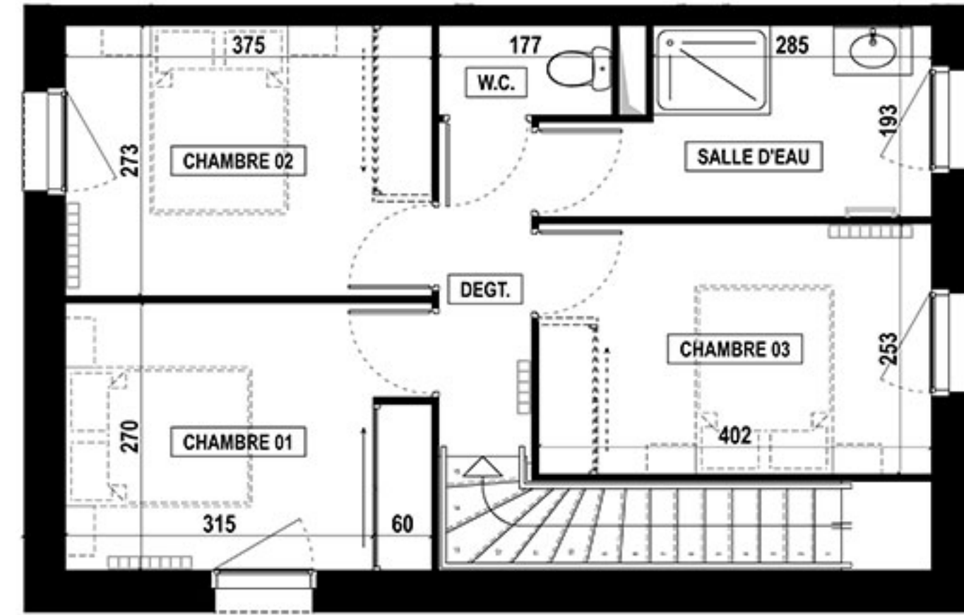
1 er ETAGE
