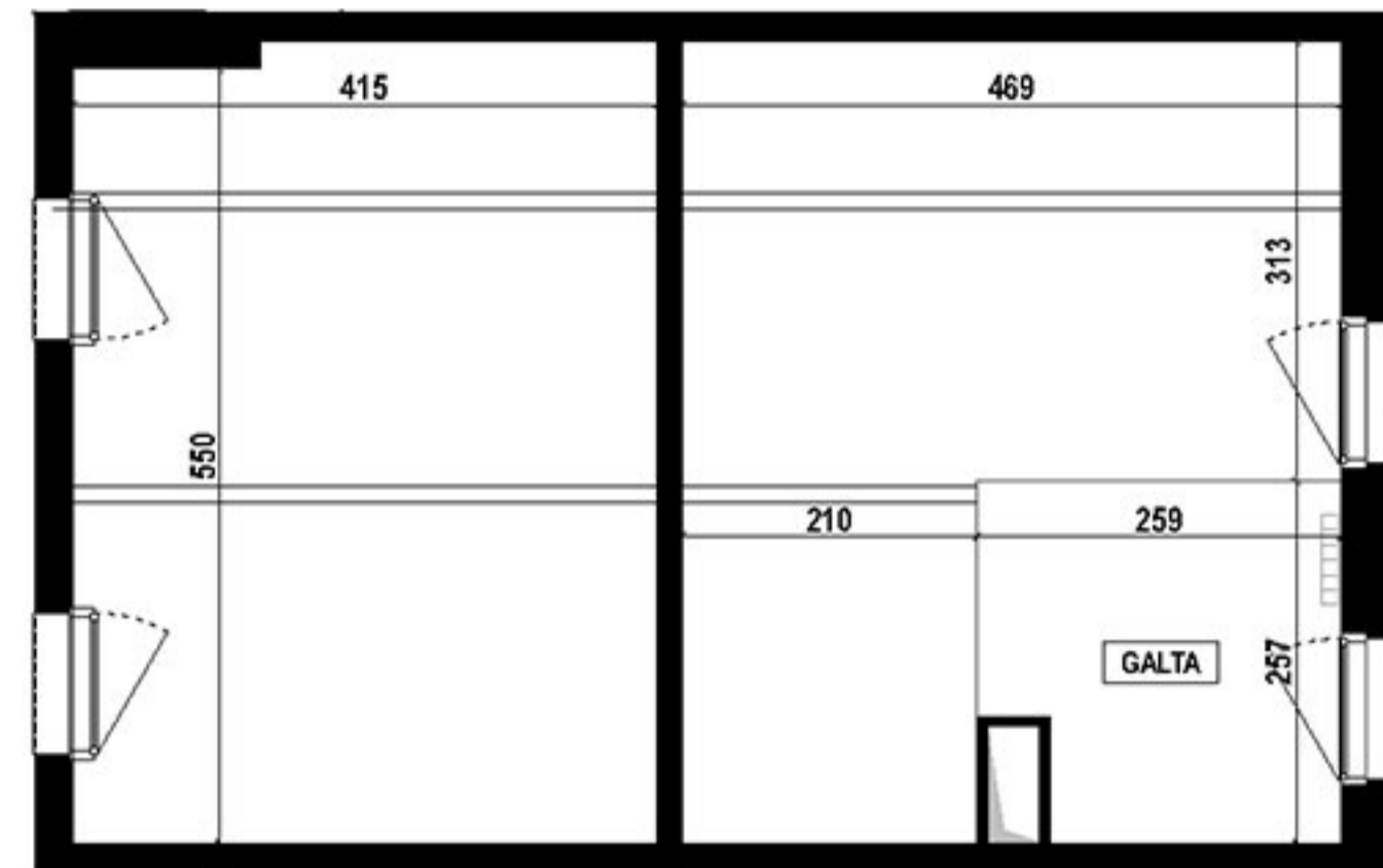
1 er ETAGE
