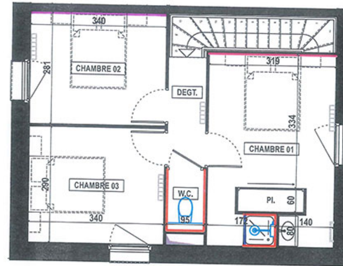
2ème ETAGE
