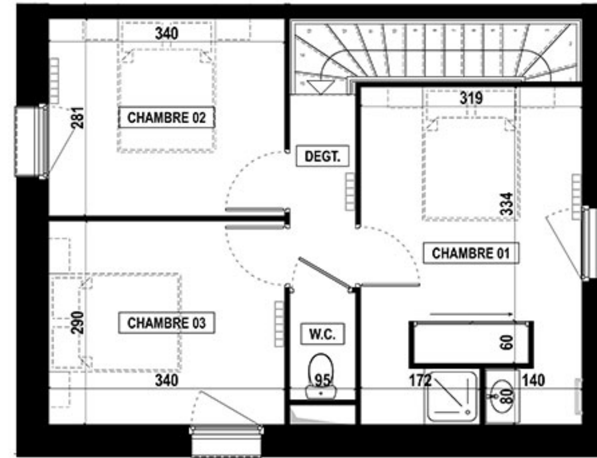
2ème ETAGE
