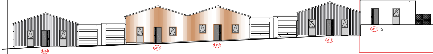
Façades NORD
