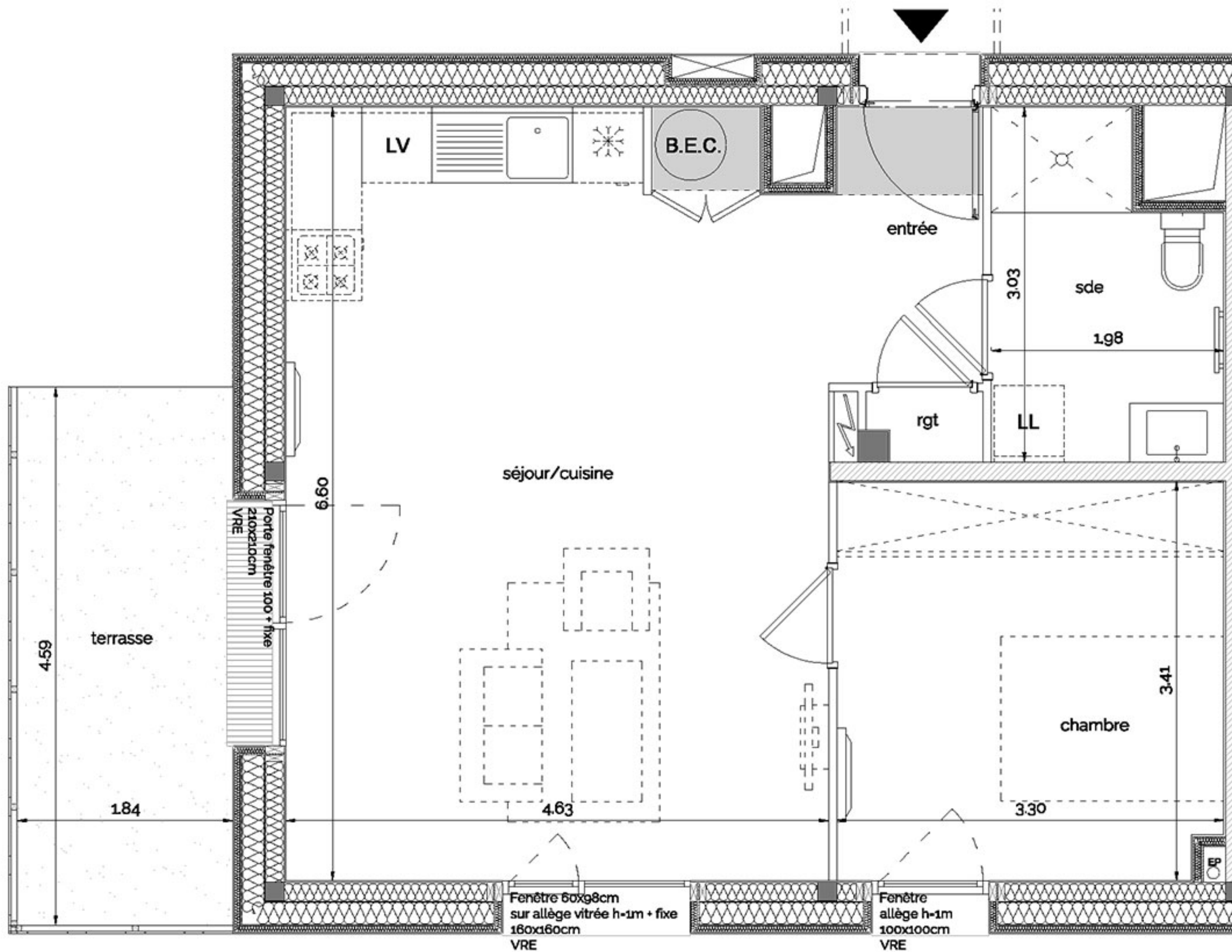
Repérage rez-de-chaussée
