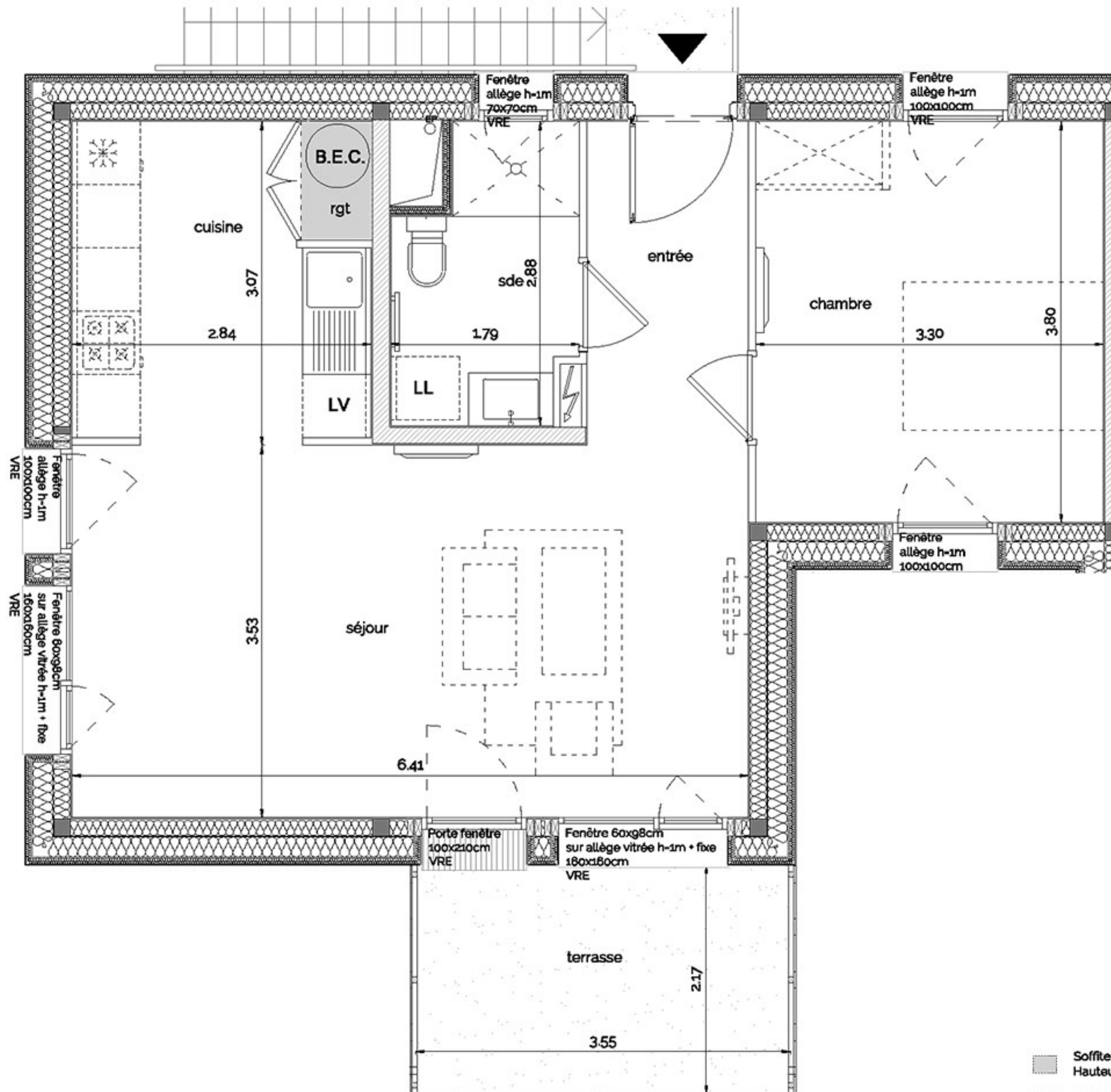
Repérage niveau 1
