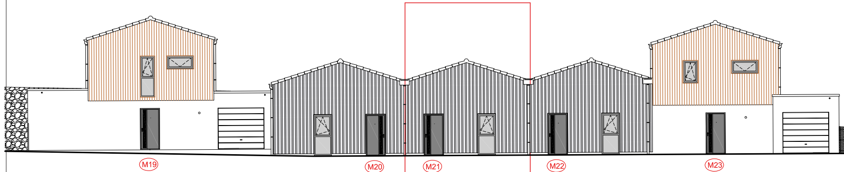
FACADES SUD-EST
