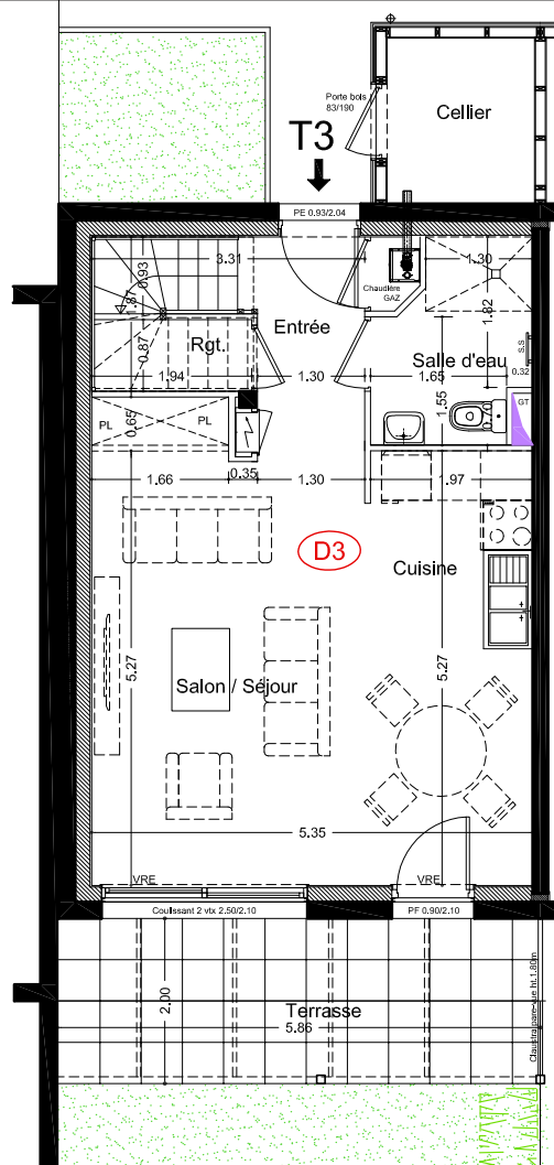
Plan Rez de Chaussée
