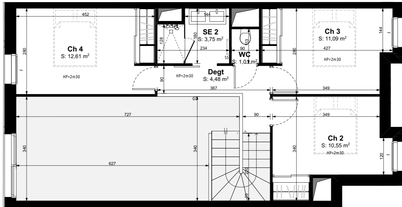
Niveau haut
