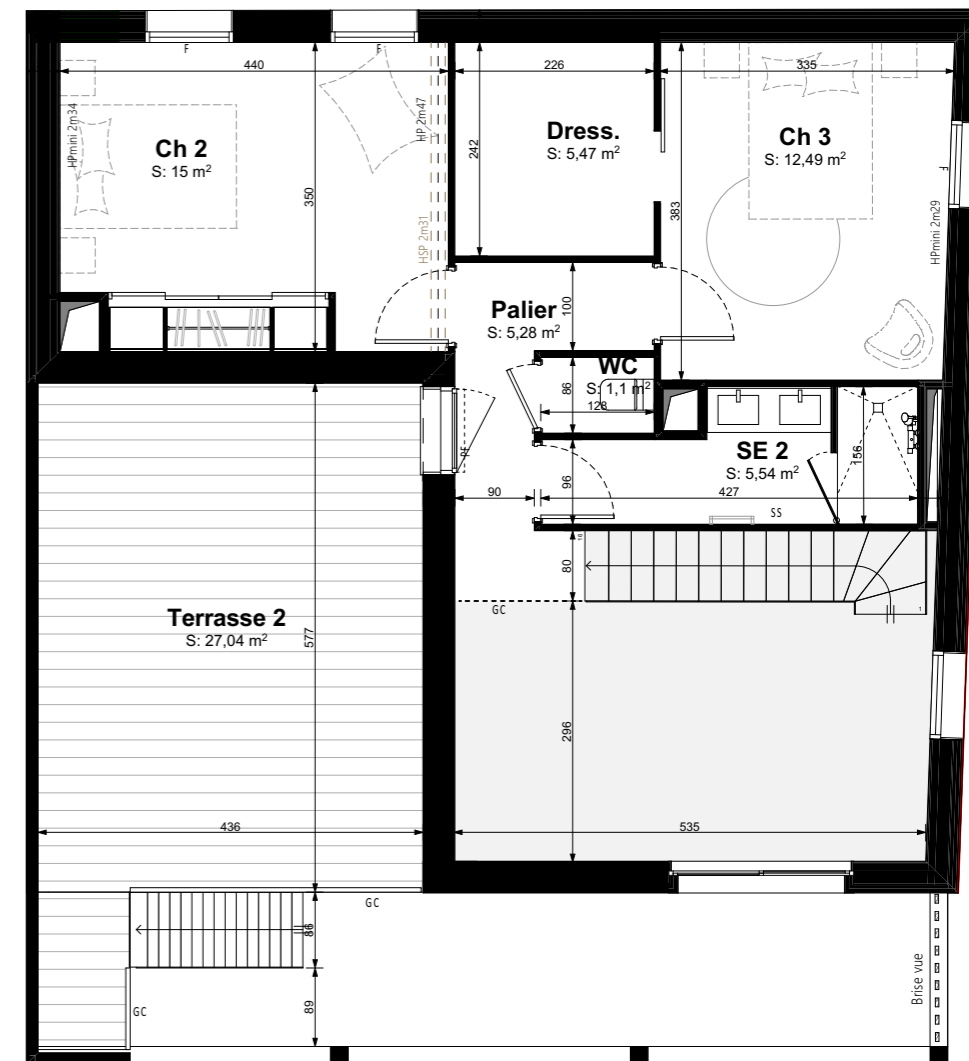
Niveau haut
